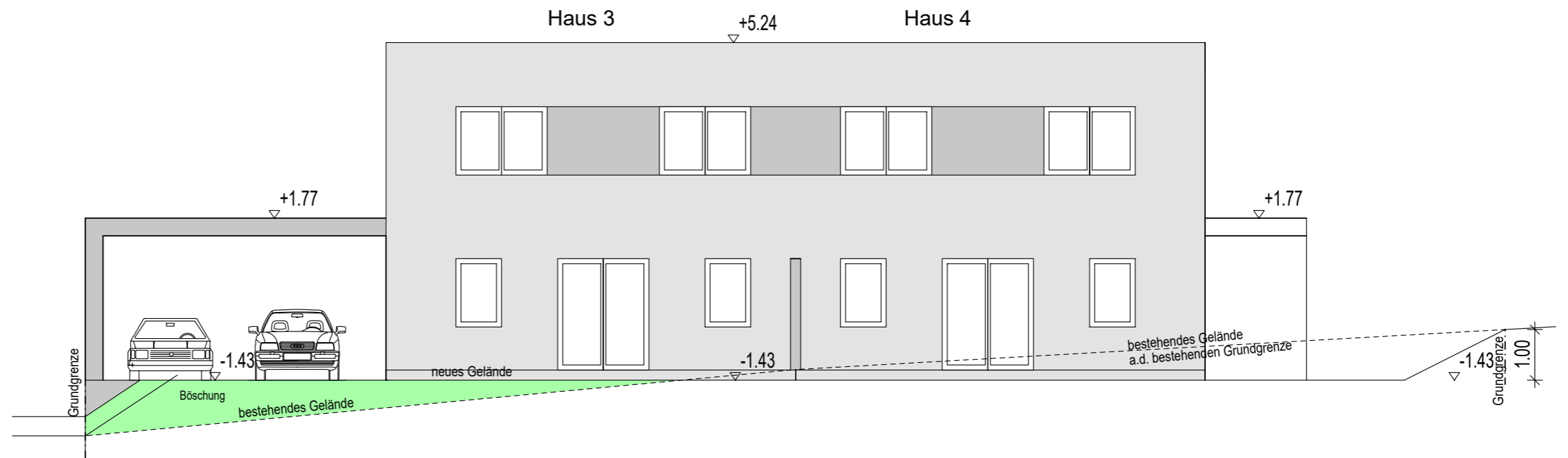
ANSICHT SÜDWEST
