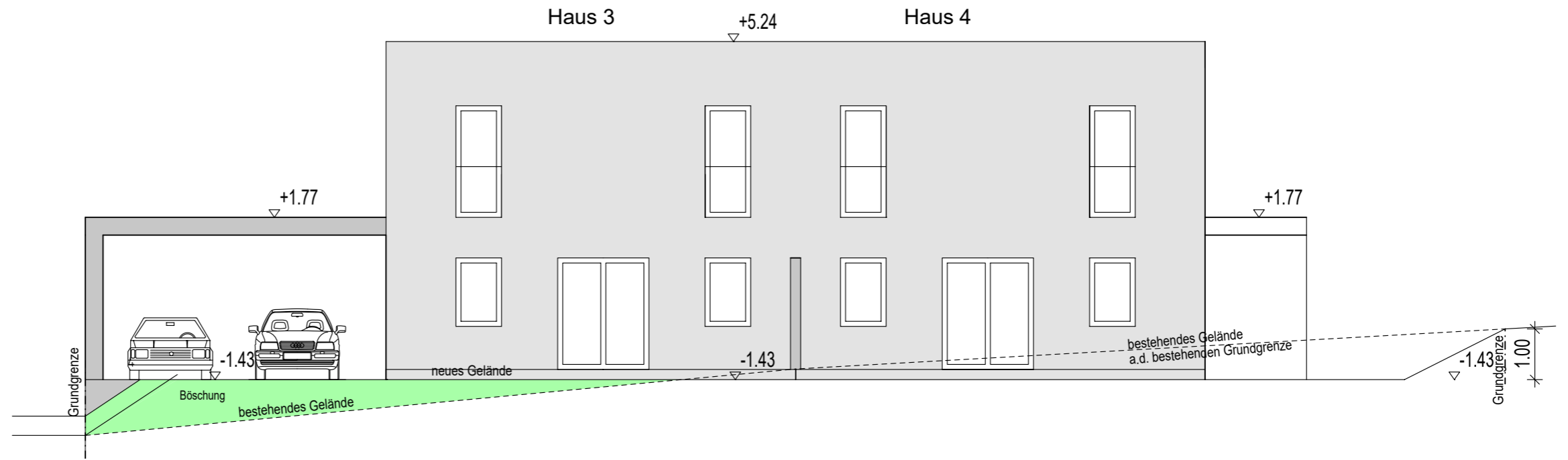
ANSICHT SÜDWEST
