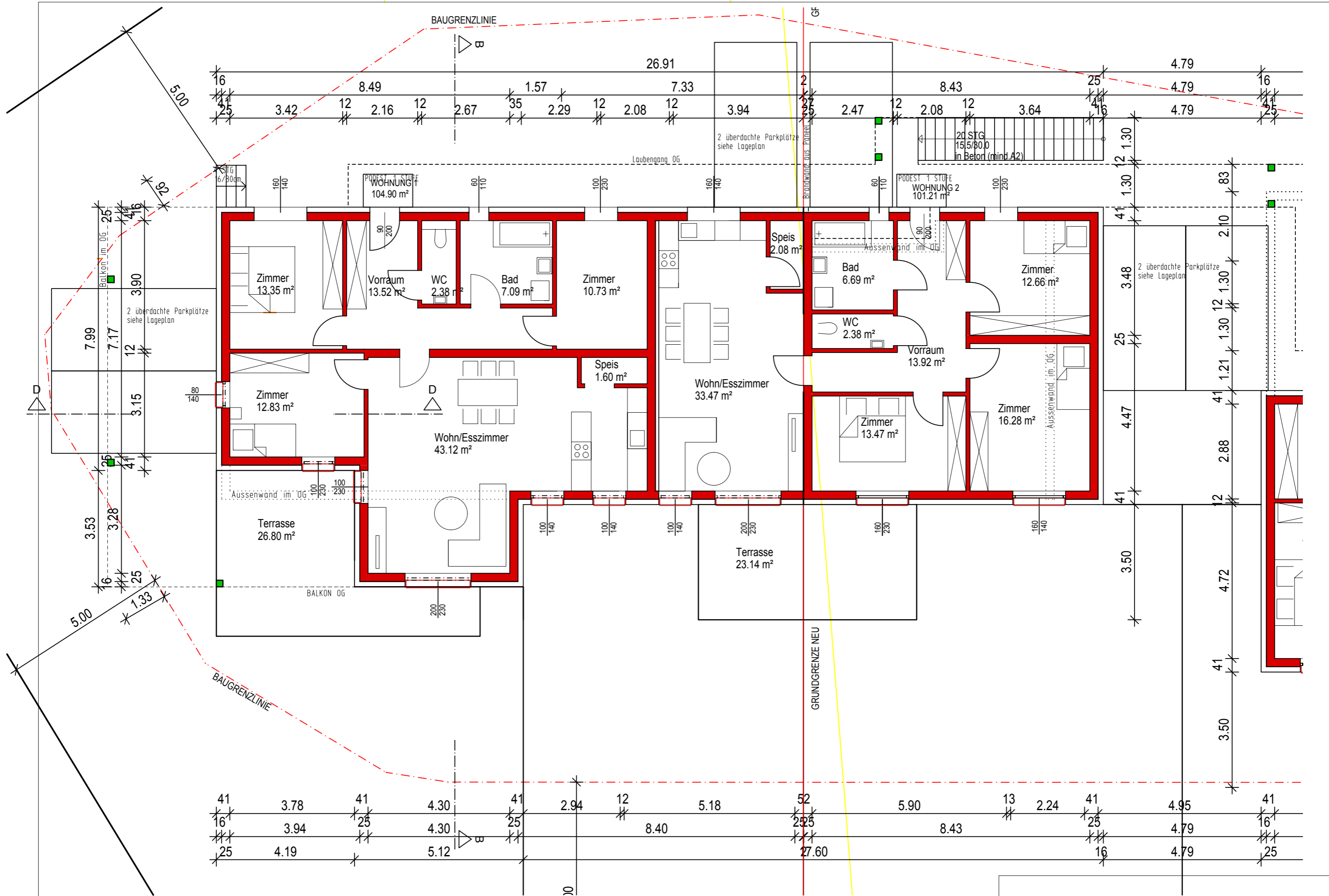
WOHNANLAGE SCHLOSSBERG VOITSBERG - GRUNDRISS ERDGESCHOSS 1:100
